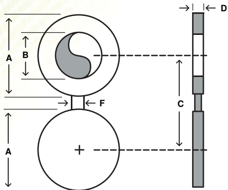
SPECTACLE BLIND TYPE 3
